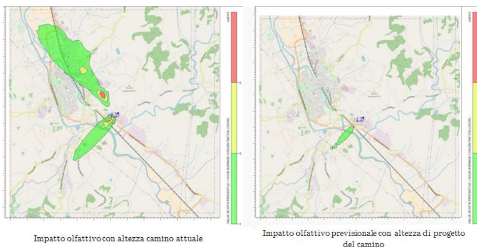
Figura 9. - Esempio di utilizzo di modellazione della dispersione atmosferica per valutazione previsionale di impatto olfattivo, a fronte dell'innalzamento del camino di emissione, da 27 a 60 metri di quota.
