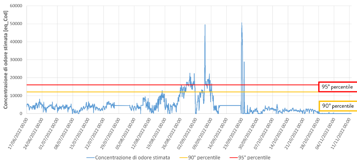
Figura 4 -3 esempio di rilevazioni quantitative operate da un IOMS installato in ingresso ad uno scrubber a servizio di un impianto di trattamento acque
