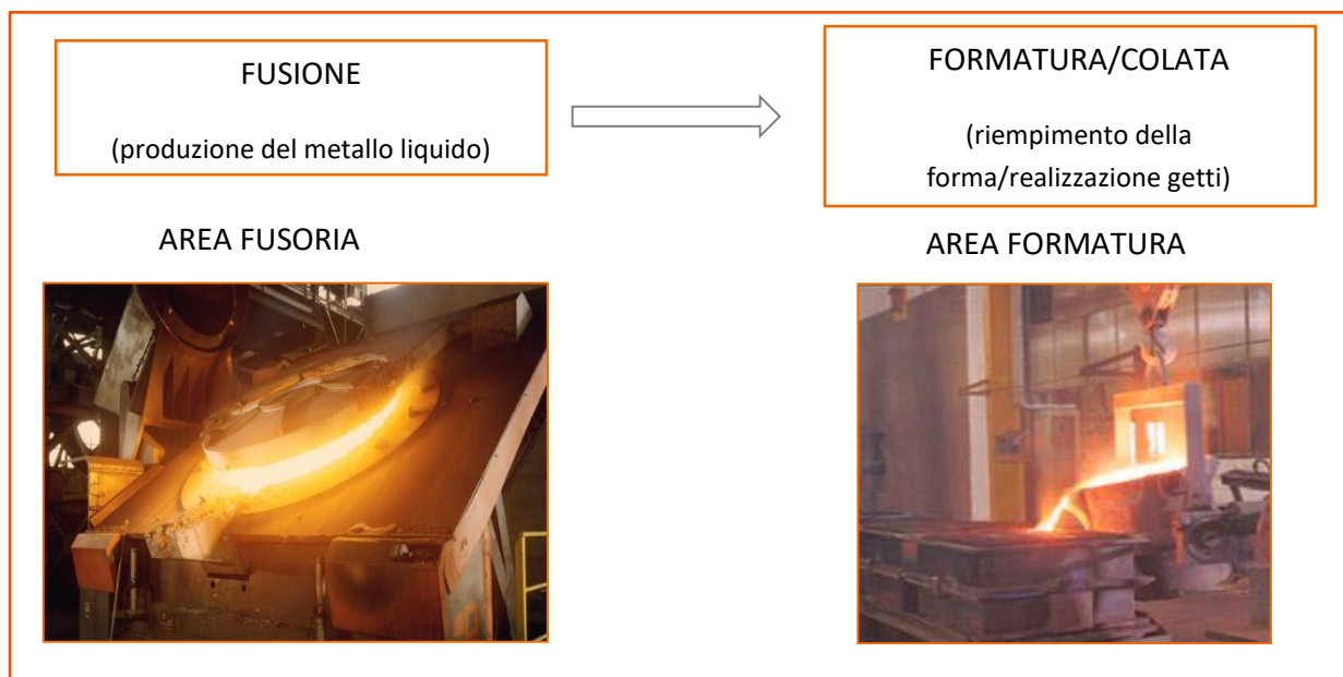
Figura 10. - Principali fasi produttive processo di fonderia
