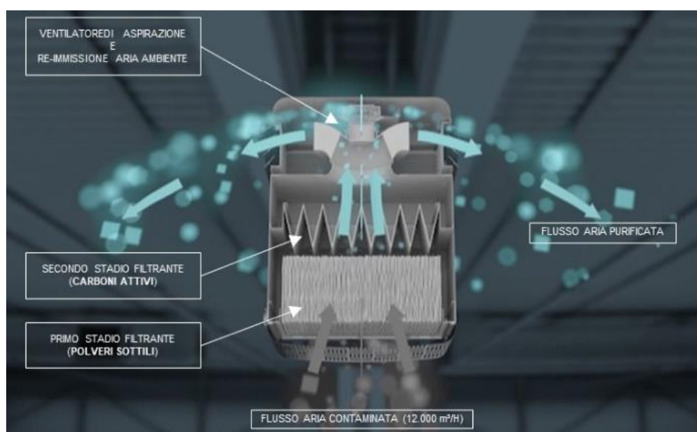
Figura 20. Schema del principio di funzionamento delle unità plug&play
