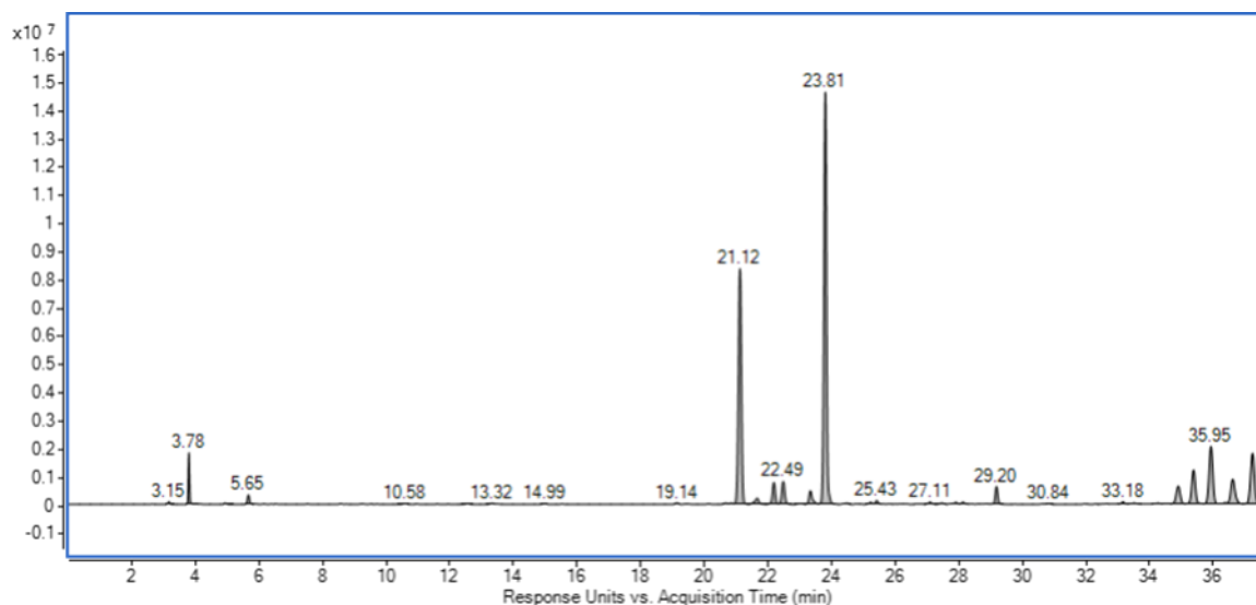
Figura 4.5 - Esempio di cromatogramma.
