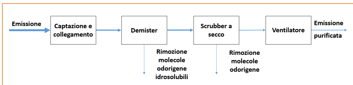
Figura 12. Diagramma a blocchi del processo di trattamento.
