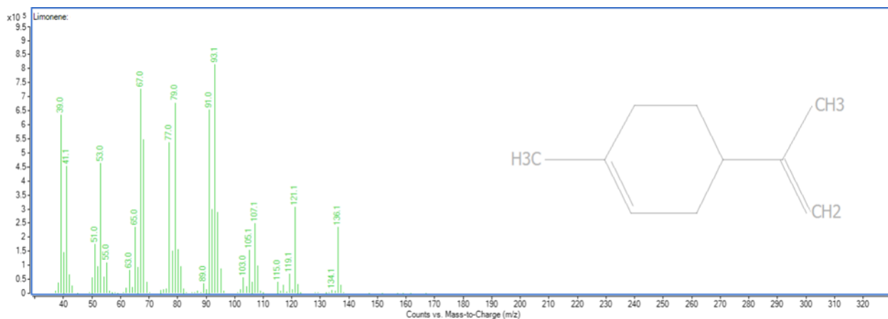
Figura 5 - Spettro di massa e relativa al picco rilevato nel cromatogramma, identificato come limonene
